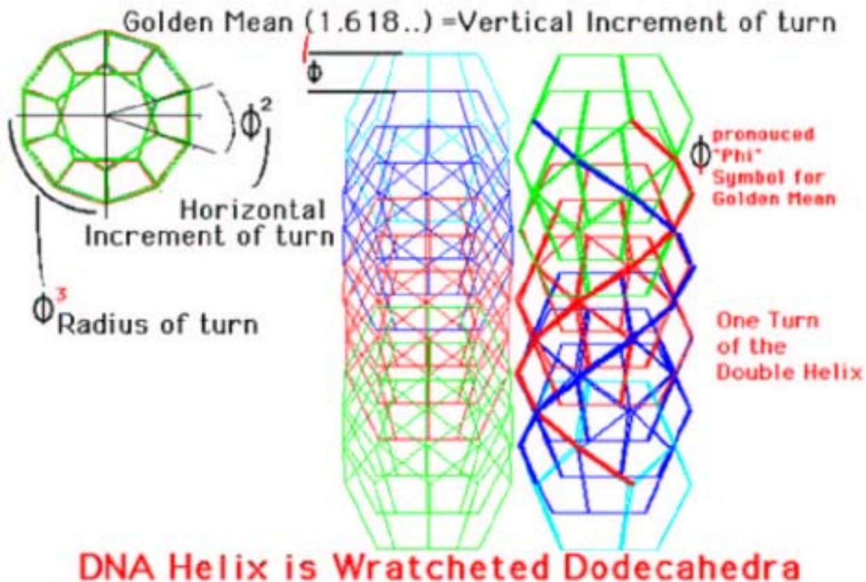
(arriba) Proporción Dorada (1.618..) = Incremento Vertical de Giro, (izq) Incremento Horizontal de giro, Radio de giro; (der.) símbolo pronunciado "Phi" para la Proporción Dorada, Un Giro de la Doble Hélice; (abajo) El ADN es un Dodecaedro "Wretcheded".
